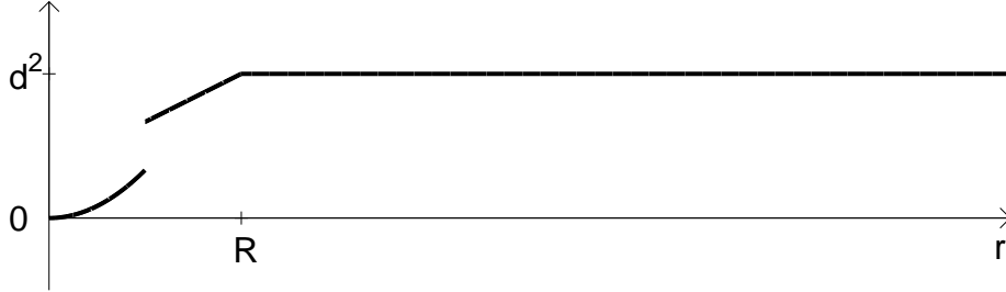
The function q(r) .
